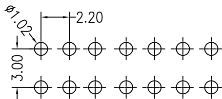
P.C.B Hole Layout
